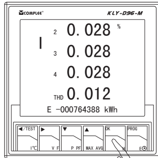
电流 2, 3, 4 次谐波及失真度
