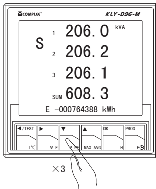
三相视在功率及总视在功率
