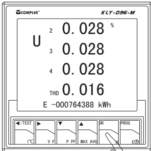
电压 2, 3, 4 次谐波及失真度
