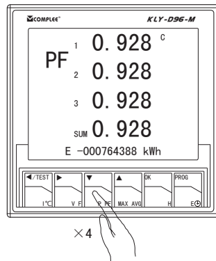
三相功率因数及总功率因数
