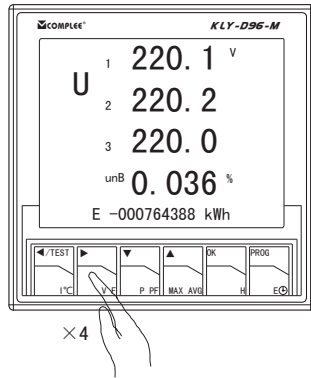
相电压及相电压不平衡度
