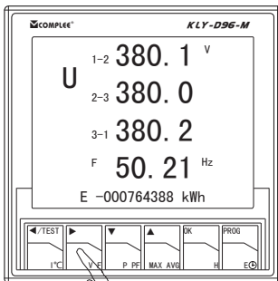
线电压及频率
