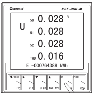
电压 50, 51, 52 次谐波及失真度
