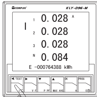
相电流及中相电流
