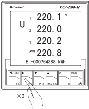
相电压及相电压平均值
