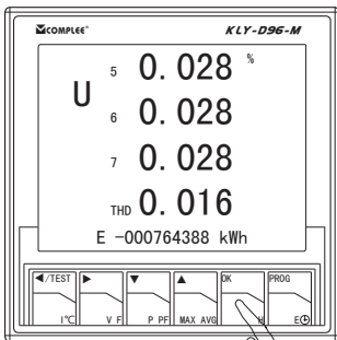
电压 5, 6, 7 次谐波及失真度
